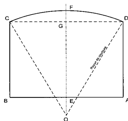
DEVELOPPEMENT PARTIE CINTRÉE
